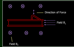
Fig. 3 The EMAT Test
